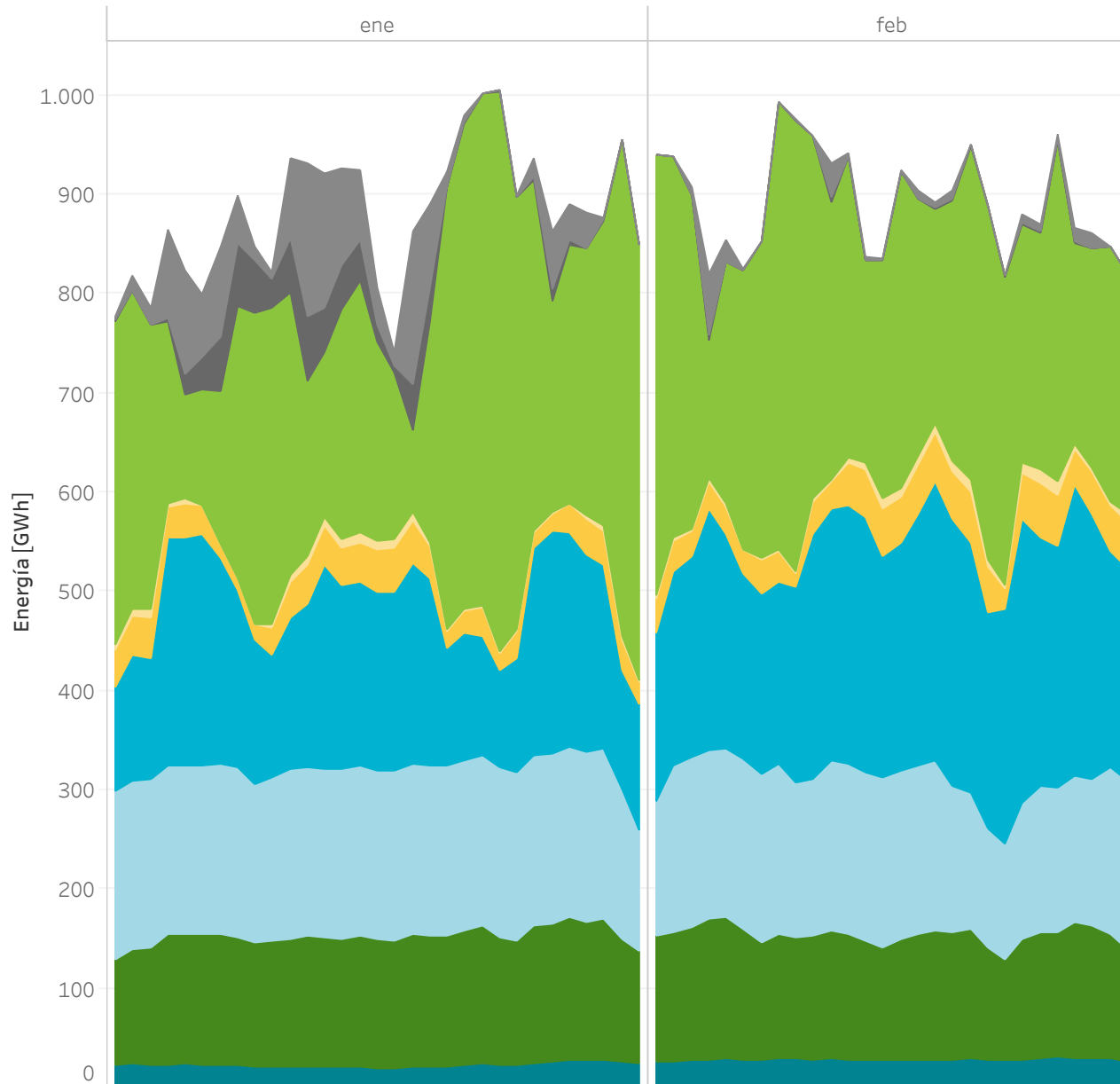
Energía por tecnologías en el Programa Diario Base de Funcionamiento (PDBF) en 2021
